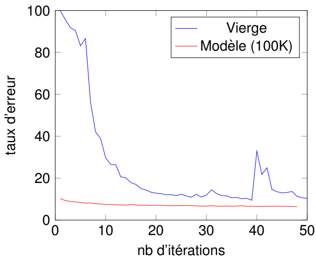
FIGURE – Amélioration de l'OCR avec modèle par défaut ou vierge
