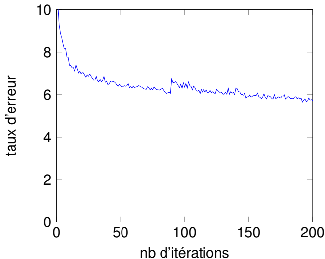
FIGURE – Amélioration du taux d'erreur de l'OCR selon le nombre d'itérations
